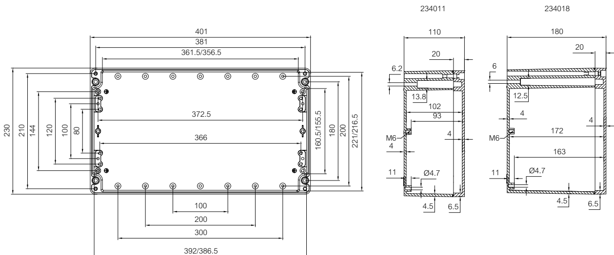
ALU 401x230x110-180
